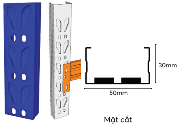
Chân Omega 50*30mm Độ dày: 0.8-1.6
