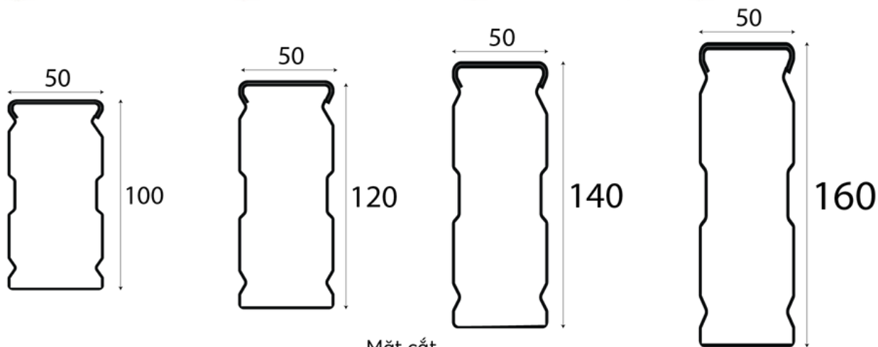
Mặt cắt
