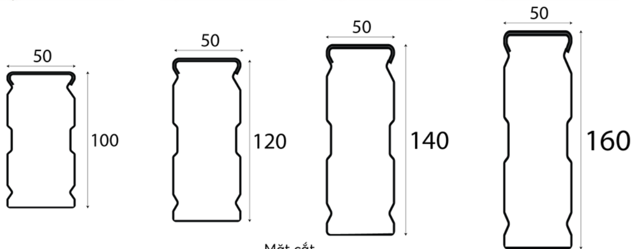
Mặt cắt
