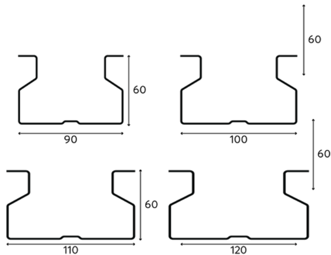
Mặt cắt
