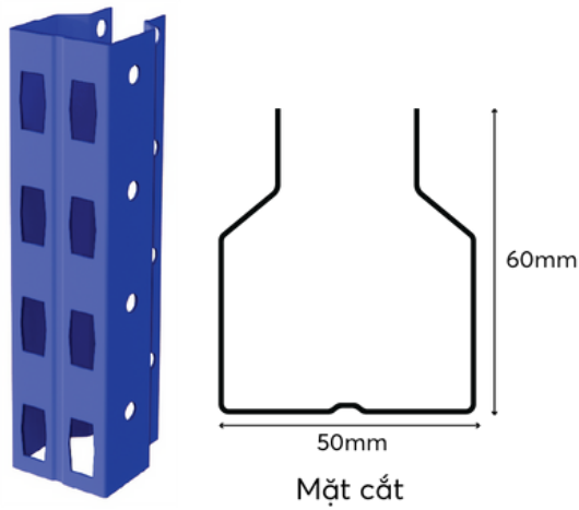
Chân Omega 50*60 Độ dày 0.8-1.6
